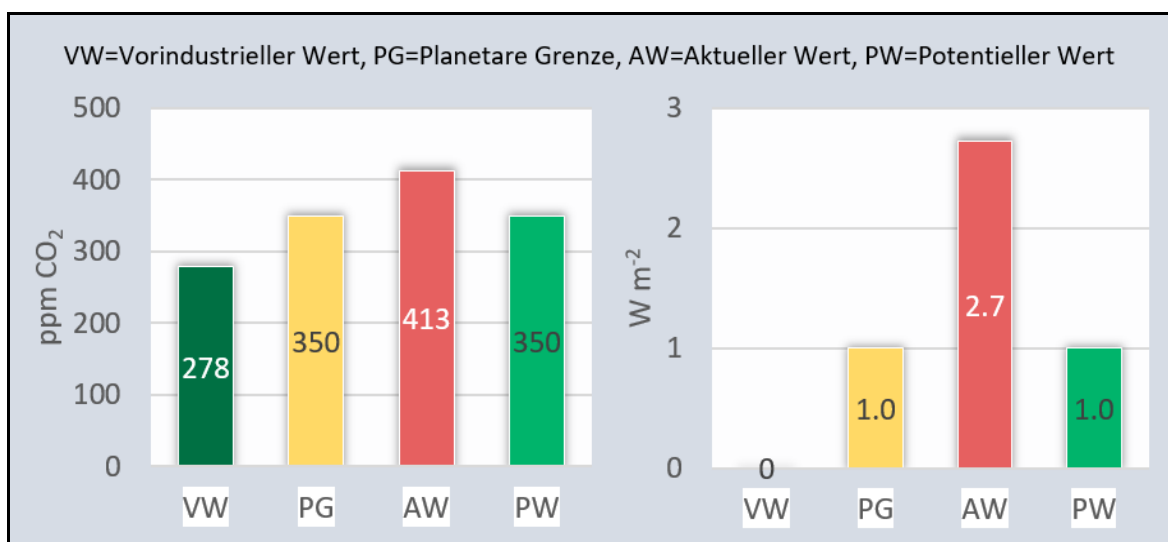
Abbildung 5: Erreichbarkeit der Planetaren Grenzen für CO 2 -Konzentration und Strahlungsantrieb mit a.) einem Wechsel auf ein pflanzenbasiertes Ernährungssystem, b.) Aufforstungen, c.) Stopp der Emissionen innerhalb von insgesamt frühestens 13 Jahren bzw. 21 Jahren
