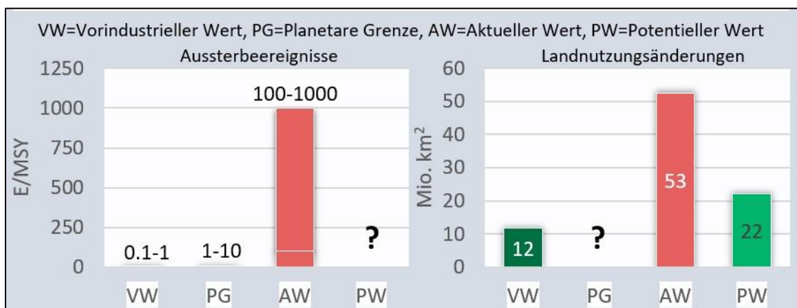
Abbildung 6: Überschreitung der Planetaren Grenze für den Verlust der Biodiversität und potentielle Reduzierung von Habitatnutzungen bei einem Wechsel auf ein pflanzenbasiertes Ernährungssystem
